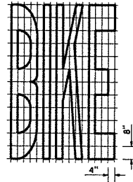
A=21 ft 2
