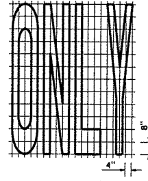
A=22 ft 2
